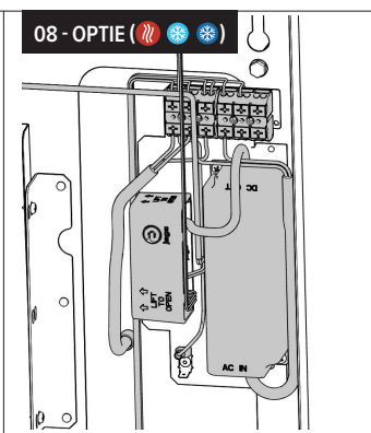
Aansluiting 230 VAC met waterdichte voeding en voorgemonteerde condenspomp met onderbrekings contact (klasse I toestel).
