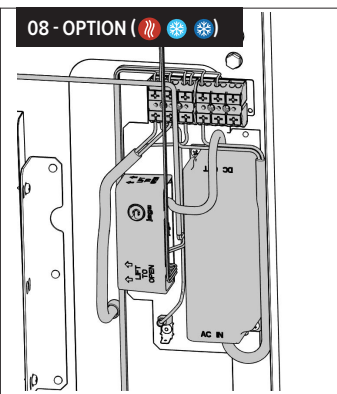
Anschluss 230 VAC mit wasserdichtem Netzteil und vormontierter Kondensatpumpe mit Trennkontakt (Klasse I Gerät).
