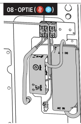
Aansluiting 230 VAC met waterdichte voeding en aansluitwartel.
