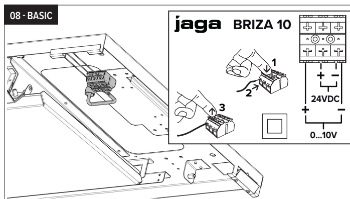
Aansluiting 24 VDC met externe sturing.
