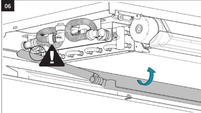
Installieren Sie den Kondensatsammler.
