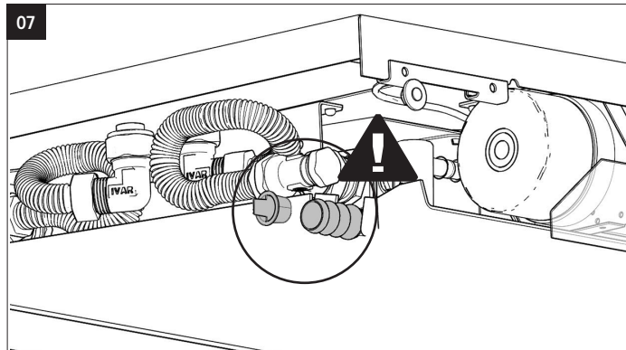
Niet-condenserend koelen - sluit de afvoernippel van de condensopvang af (Ø2cm).
