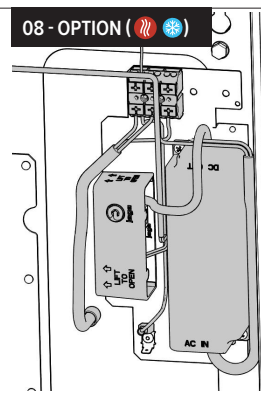
Anschluss 230 VAC mit wasserdichtem Netzteil und Anschlussklemme.
