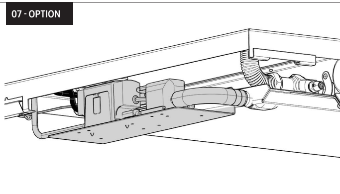
Kondensierende Kühlung - vormontierte Kondensatpumpe mit Trennkontakt (Gerät der Klasse I).
