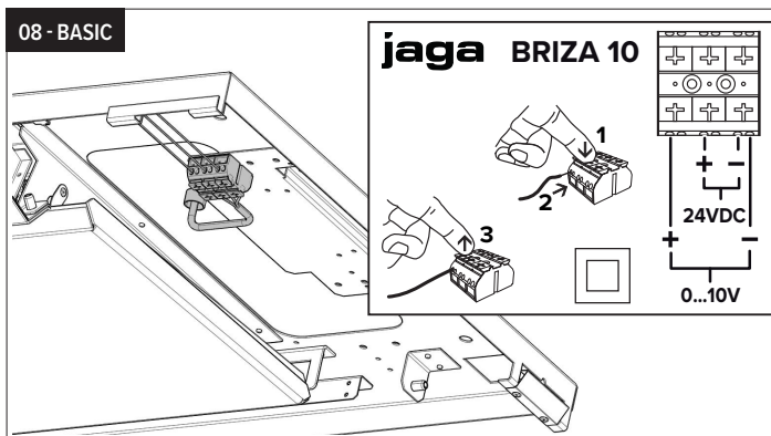
Anschluss 24 VDC mit externer Steuerung.
