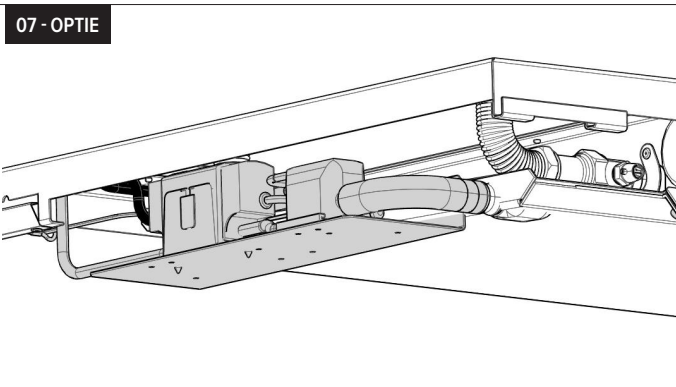
Condenserend koelen - voorgemonteerde condenspomp met onderbrekings contact (klasse I toestel).
