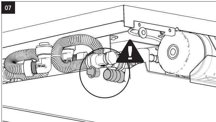
Nicht-kondensierende Kühlung - Ablaufanschluss des Kondensatsammlers muß verschlossen werden (Ø2cm).
